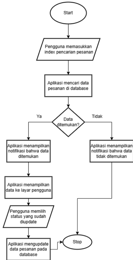
Gambar 4. Flowchart fitur “konfirmasi pesanan”
