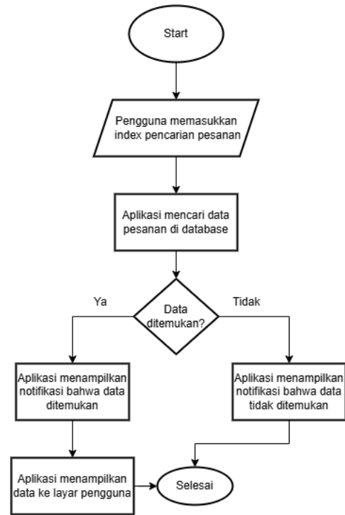
Gambar 3. Flowchart fitur “lihat pesanan”
